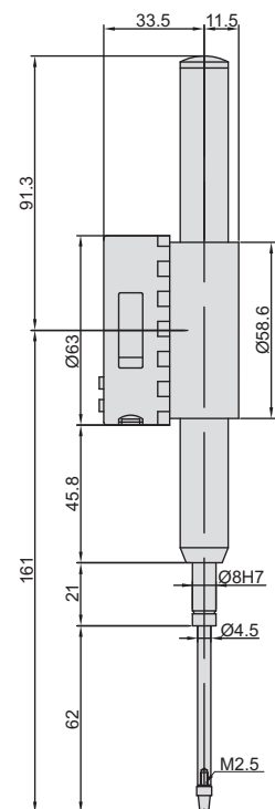
Range: 0-50.8mm
